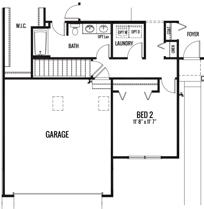
OPTIONAL BASEMENT
